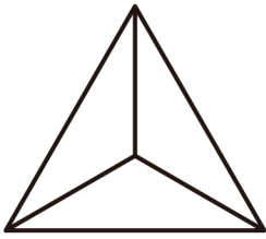
正四面體
