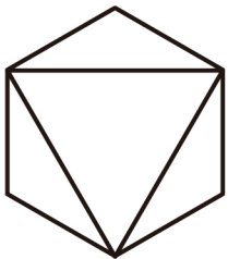
正八面體
