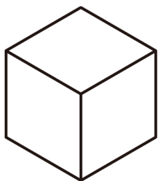
正六面體
